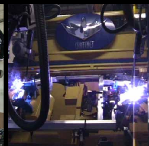
Soudure du châssis par double robot
